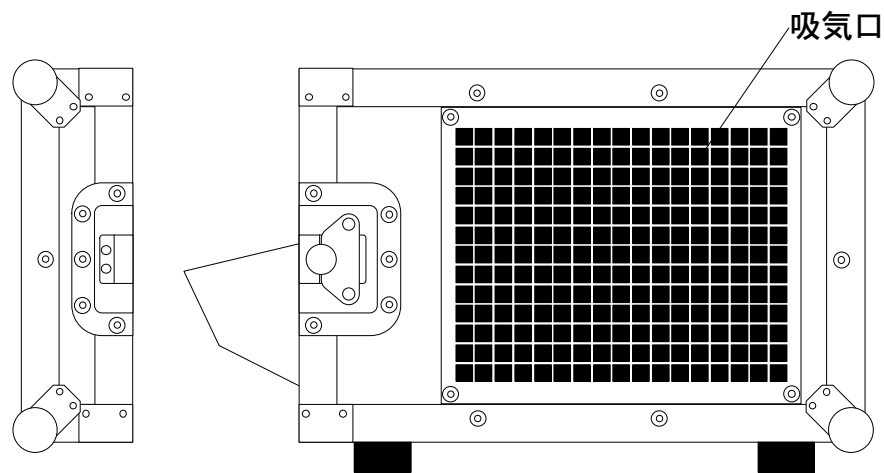
側面図
