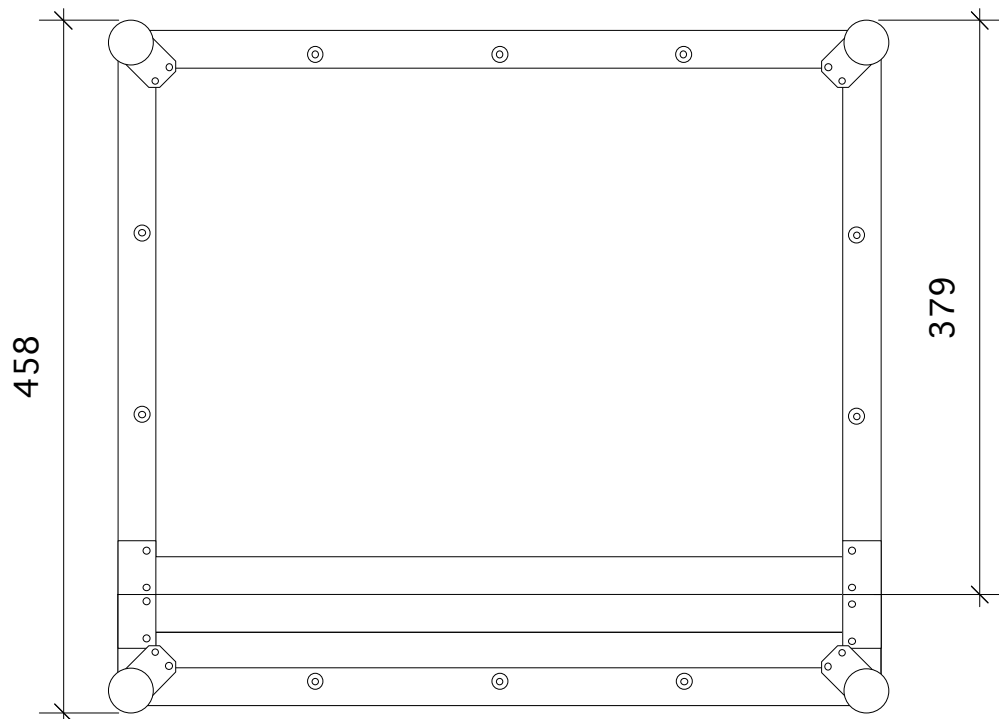
上面図
